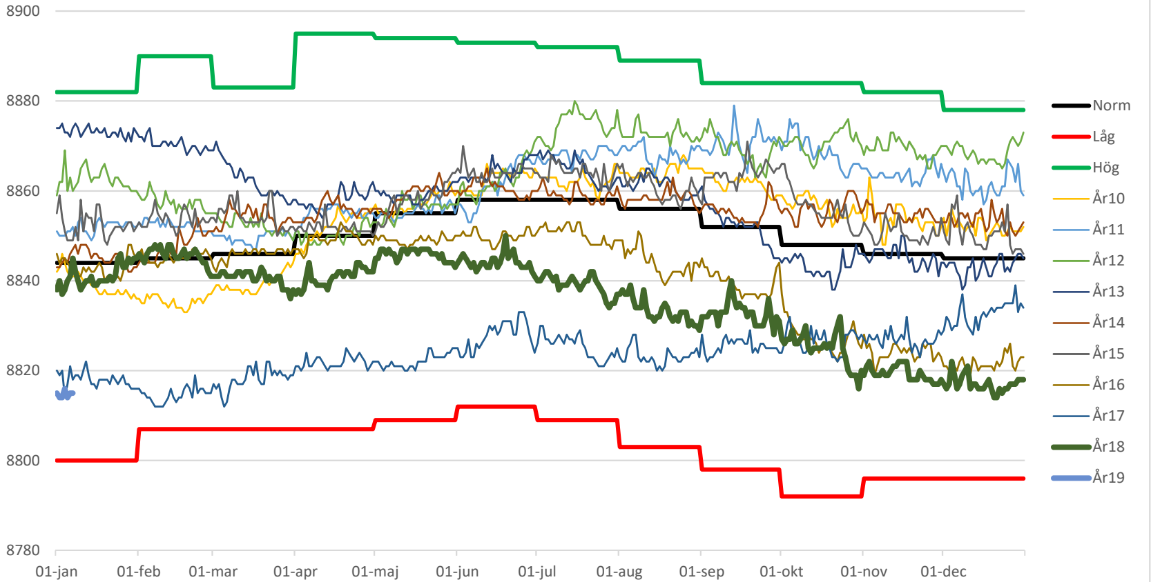
Vättern vattenstånd 2010-2019
